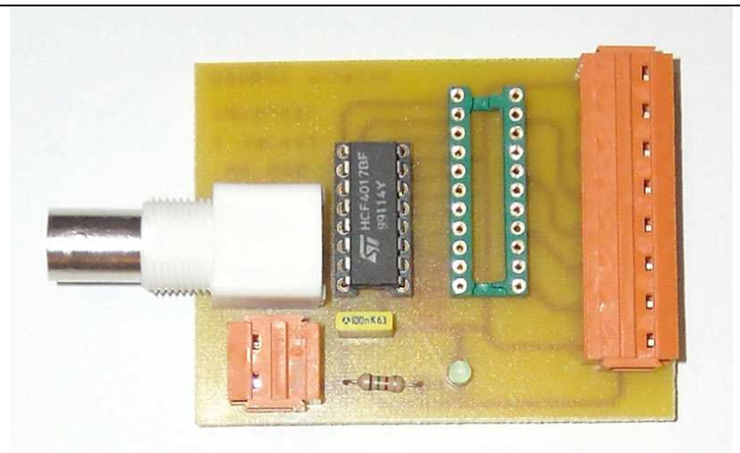
Figure 2.10. Vue de la carte électronique (images-maquettes\TESTEUR1-12.jpg).
