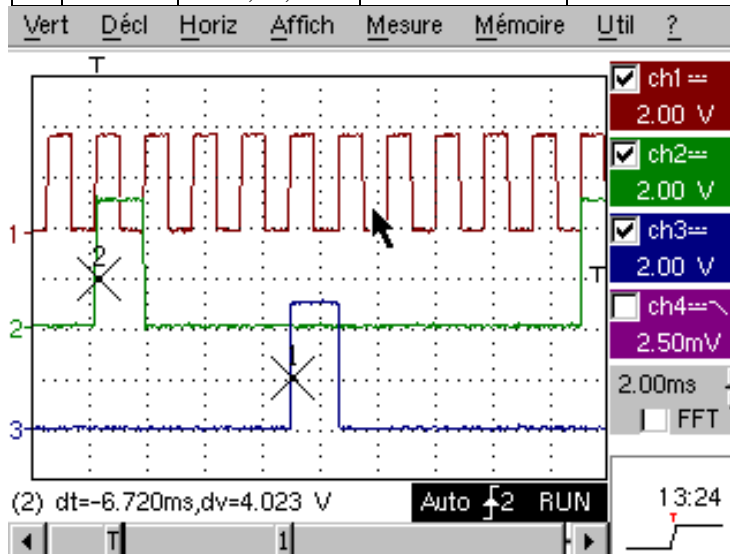
Figure 2.11. Chronogramme de fonctionnement (TESTEUR1.gif).
