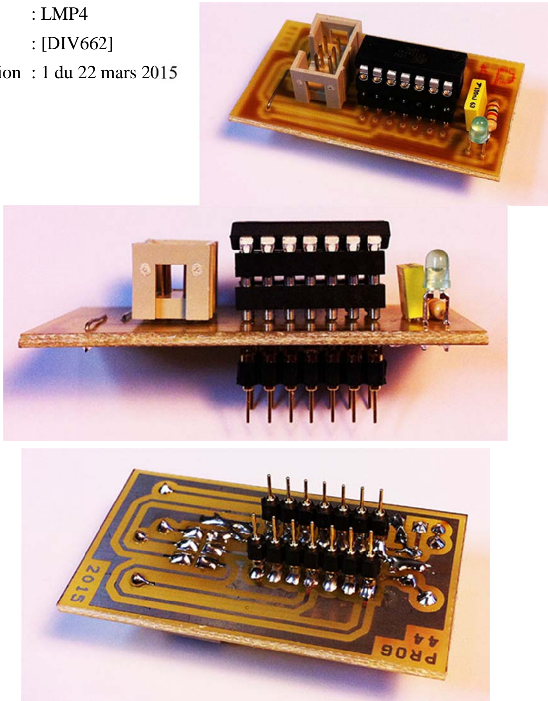
Fig. 12.7. Vue d'ensemble du montage (images-composants\PROG44-12, 22 & 32.jpg).
