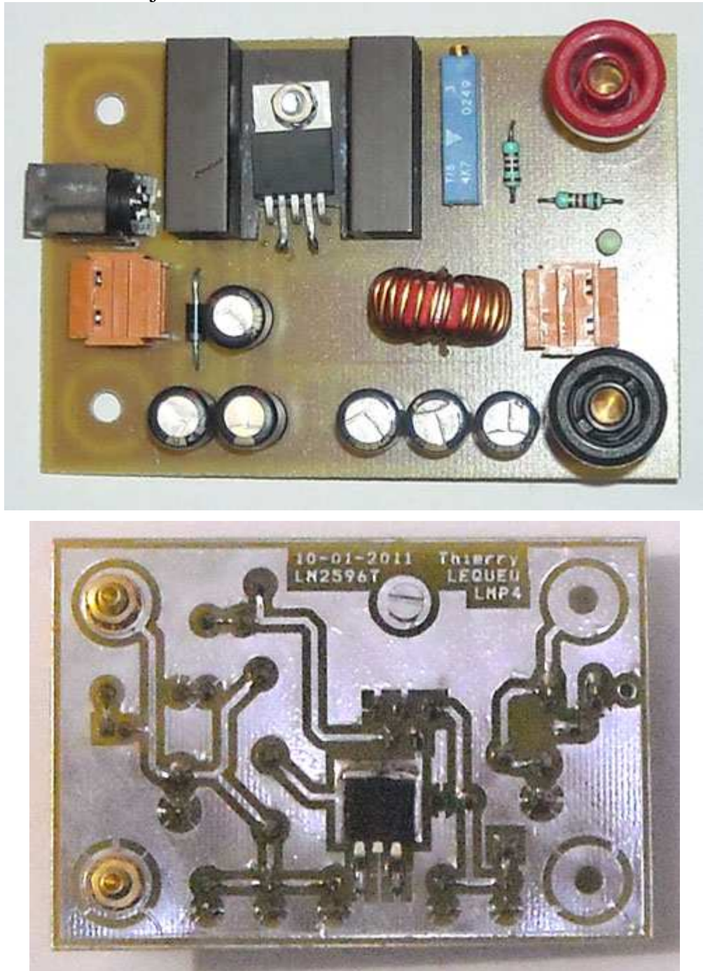
Fig. 5.6. Vue d'ensemble du montage (images-composants\LM2596T-13 & 23.jpg).
