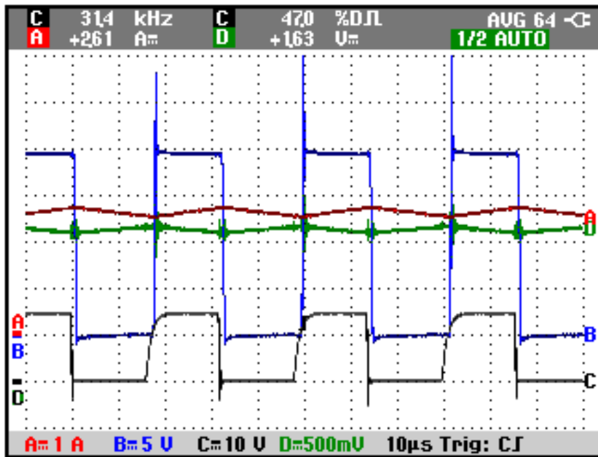
Fig. 11.11. Courant de l'inductance et tension de sortie du capteur de courant (2014-02-06-Mesures\2014-02-07-H2Q-B-1.bmp).
