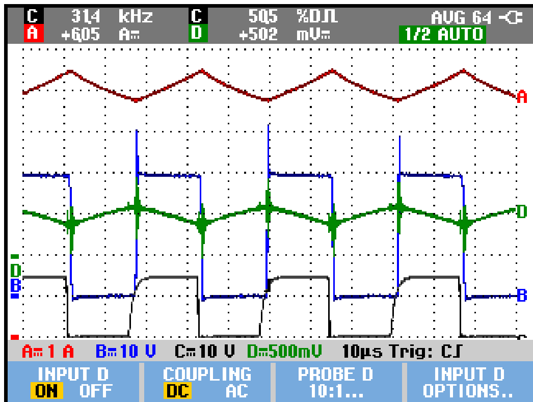
Fig. 11.12. Courant de l'inductance et tension de sortie du capteur de courant (2014-02-06-Mesures\2014-02-07-H2Q-B-2.bmp).
